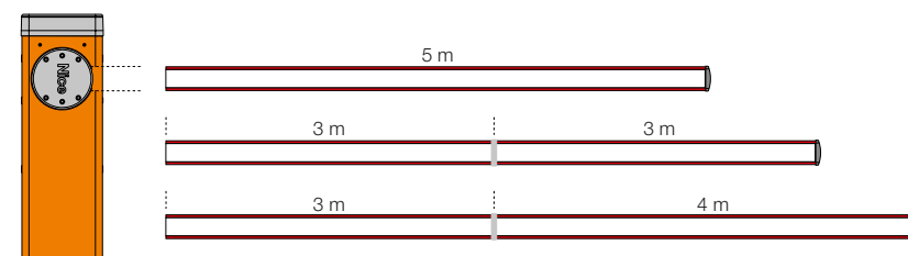
M7BAR Met boom van 5 m Uitgerust voor: beschermend rubber, sig- naleringslichten, rek (2 st.), mobiele steun Met boom van 6 m (3+3 m)* Uitgerust voor: beschermend rubber, signaleringslichten, rek (2 st.), mobiele steun Met boom van 7 m (3+4 m)* Uitgerust voor: beschermend rubber, signaleringslichten, mobiele steun
